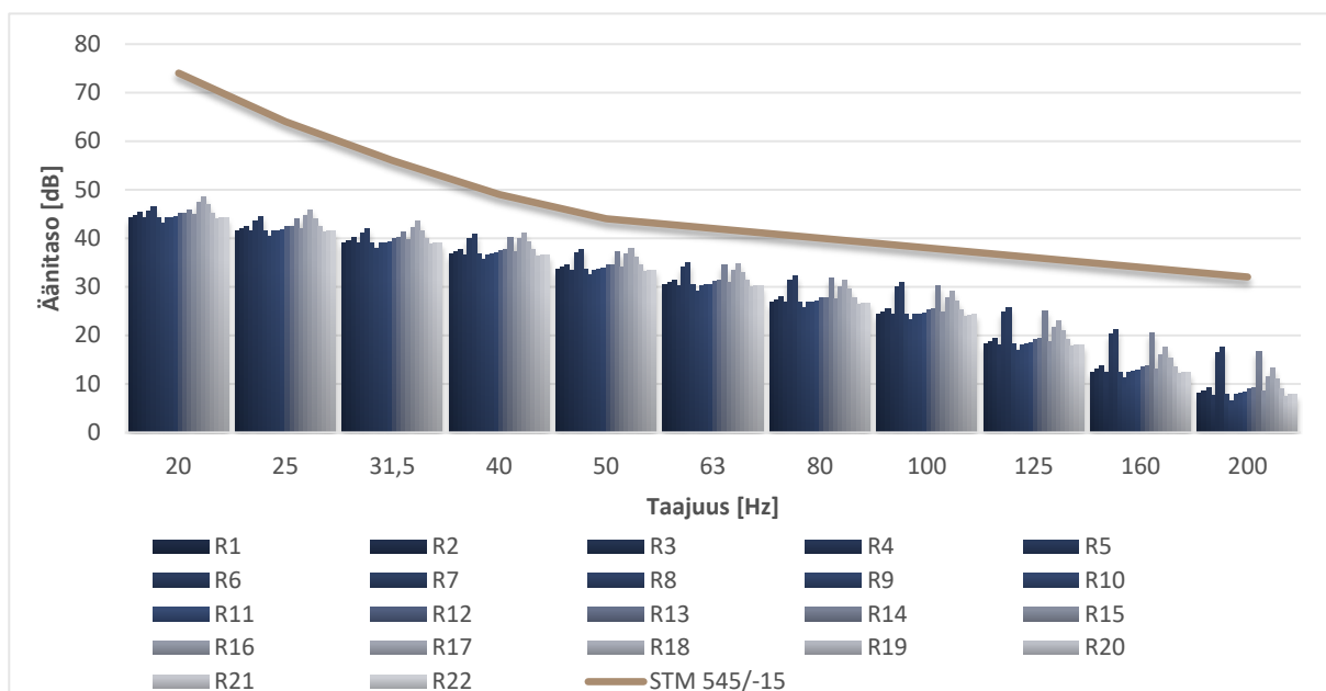
Kuva 3-2. Osayleiskaavasuunnitelman mukaisen pientaajuisen melulaskennan tulokuvaaja
