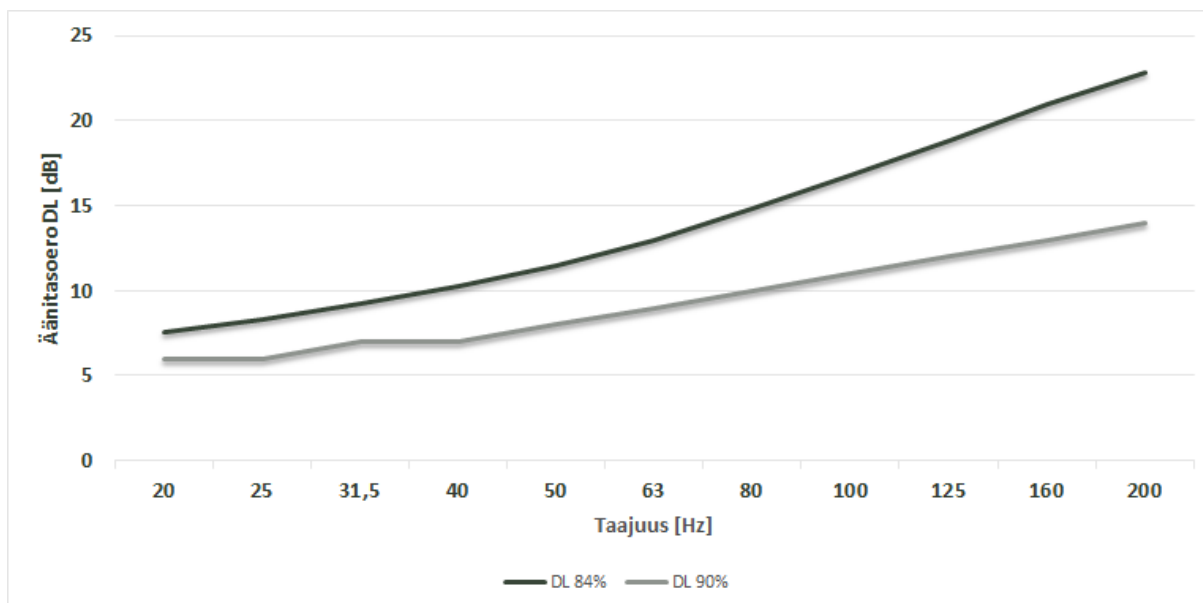
Kuva 2-3. Äänitasoeron DL vähimmäisarvon estimaatit 85% ja 90% persentiileille Turun AMK:n julkaisujen mukaan (Keränen, 2017, 2019).
