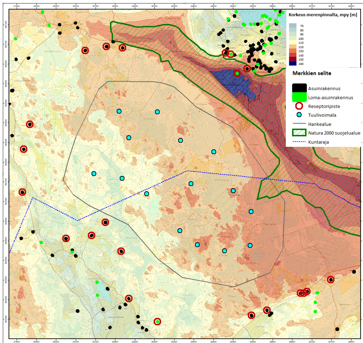
Kuva 2-1. Melumallinnuksen digitaalikartan topografiamalli, mpy [m]
